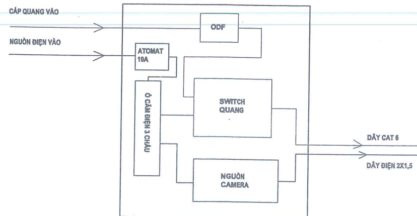
SƠ ĐỒ ĐẦU NỐI TỪ CAMERA
