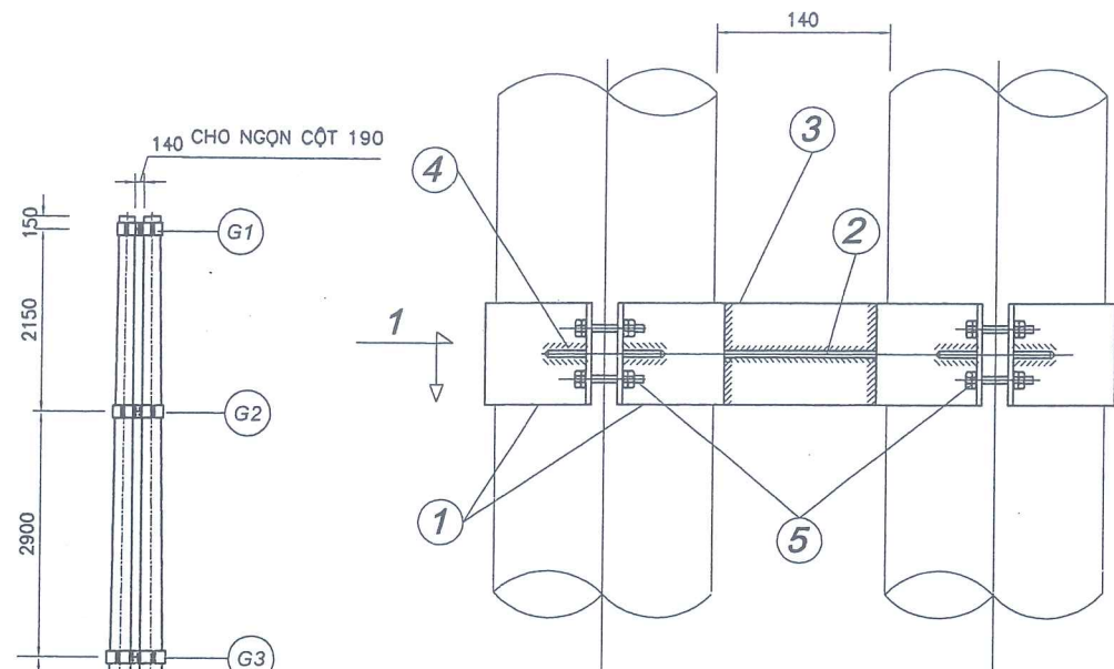
MẶT CHÍNH
