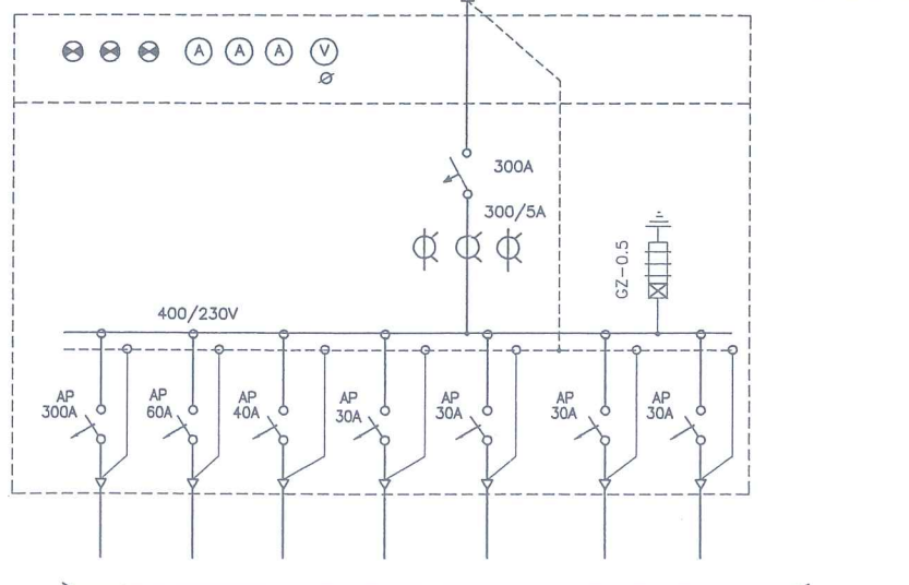
SƠ ĐỒ NỐI ĐIỆN CHÍNH CỦA TỦ PP ĐIỆN TỰ DÙNG
