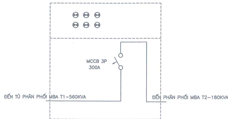
SƠ ĐỒ NỐI ĐIỆN CHÍNH CỦA TỦ PHÂN ĐOẠN MBA T1 VÀ T2
