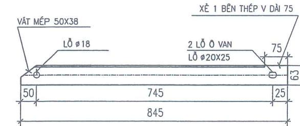
CHI TIẾT THANH CHỐNG ②B TỶ LỆ 1:10
