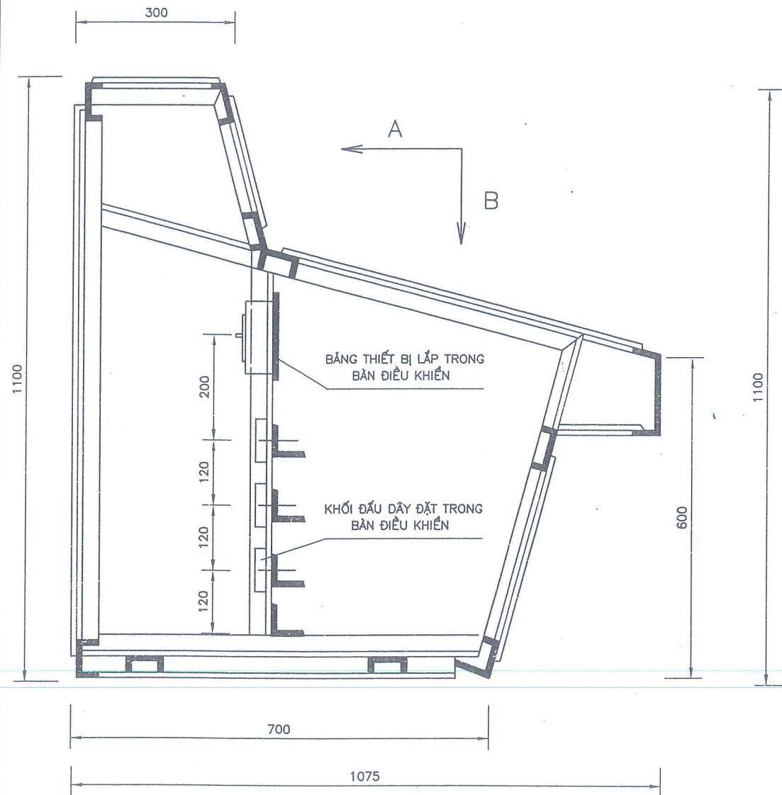
NHÌN THEO C-C (TỈ LỆ: 1/10)
