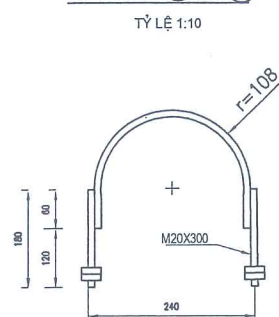
CHI TIẾT ⑤ VÀ ⑥
