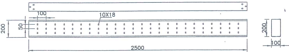
CHI TIẾT MÁNG CÁP 200X100
