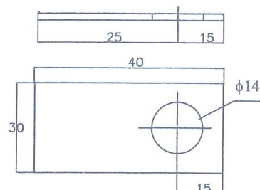
6-LỖ LUỒN BU LÔNG KEP CHÌ
