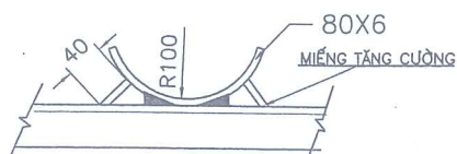
CHI TIẾT ÔM CỘT TỶ LỆ 1:20
