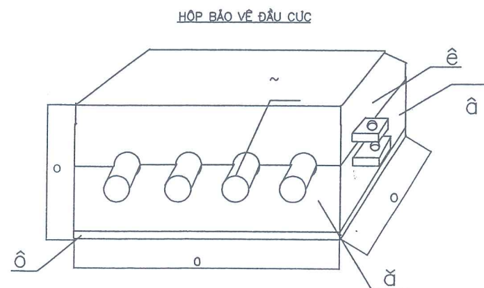
2-THÂN HỒM
