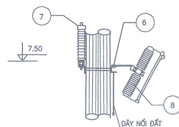
MẶT NGHIÊNG
