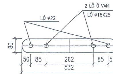
THANH BẮT CHUỖI ④ TỶ LỆ 1:10
