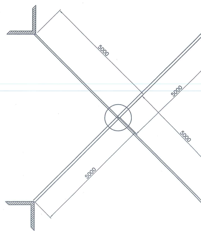
MẶT BẰNG BỐ TRÍ CỌC TIẾP ĐỊA TỶ LỆ 1:250
