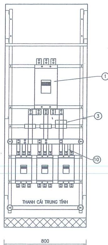
SƠ ĐỒ NỐI ĐIỆN CHÍNH CỦA TỦ MBA 560KVA
