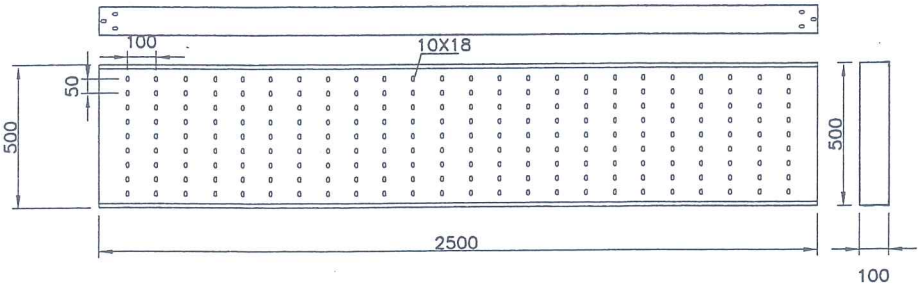
CHI TIẾT MÁNG CÁP 500X100
