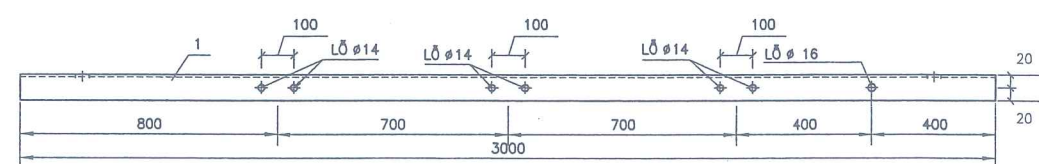
THANH XÀ BẮT CẦU CHỈ TỰ RƠI
