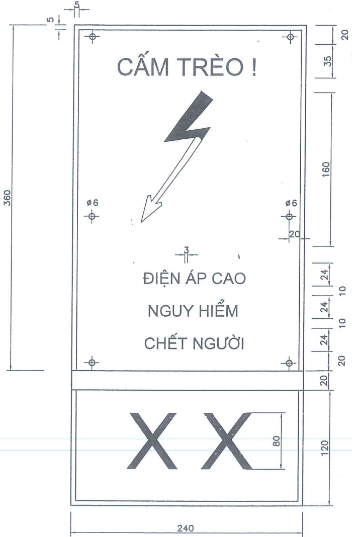
BẢNG NGUY HIỂM-SỐ TRỤ TOLE TRẮNG KÈM 0,8X240X480
