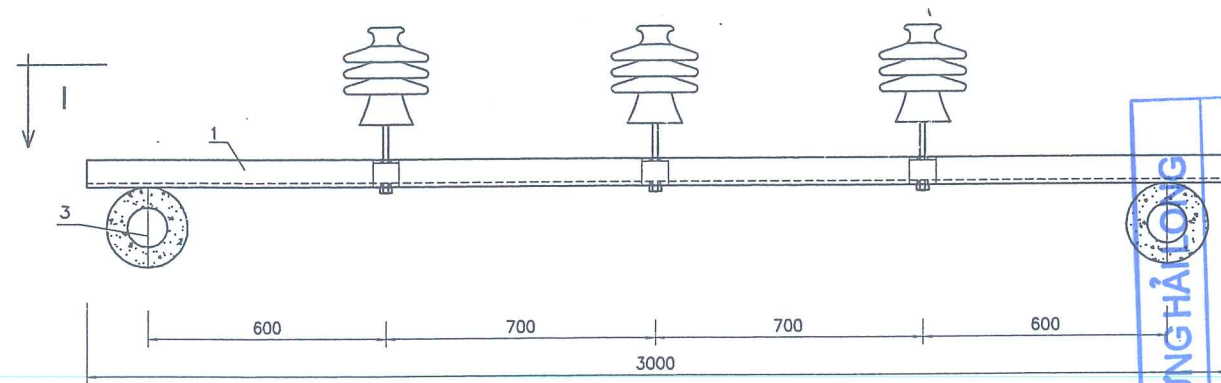
MẶT BẰNG TỈ LỆ 1:20
