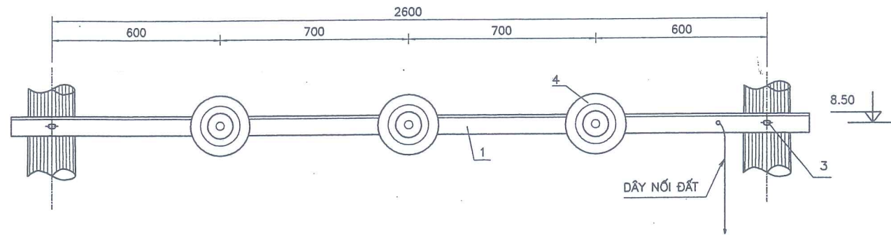
MẶT BẰNG TỈ LỆ 1:20
