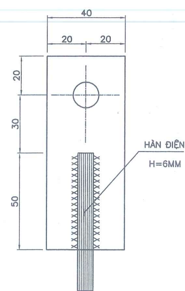
BẢN NỐI ĐẤT TỶ LỆ 1:2
