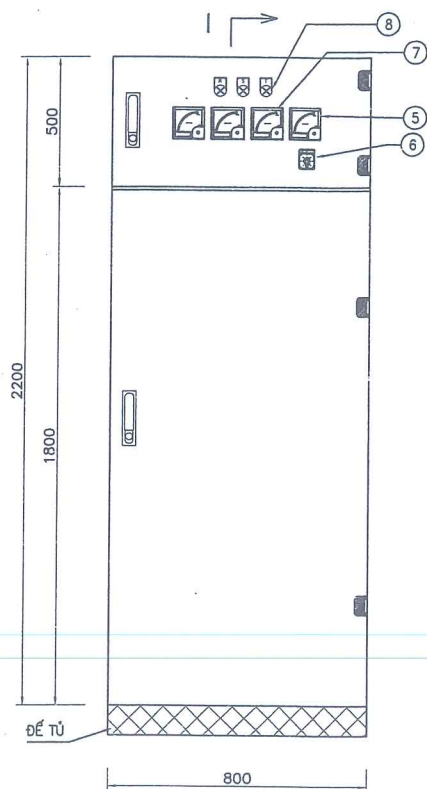
MẶT TRƯỚC
