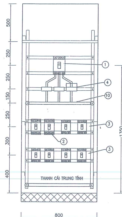
SƠ ĐỒ NỐI ĐIỆN CHÍNH CỦA TỦ PP ĐIỆN TỰ DÙNG
