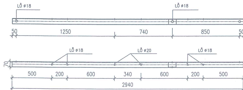
CHI TIẾT THANH XÀ CHÍNH ① TỶ LỆ 1:25
