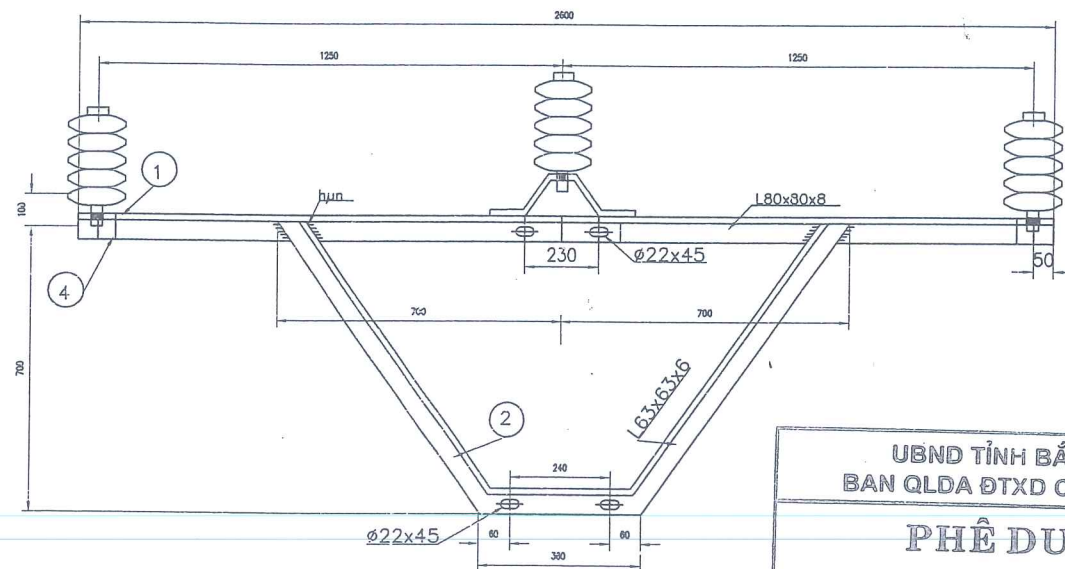
MẶT ĐÚNG XÀ TỶ LỆ 1:20
