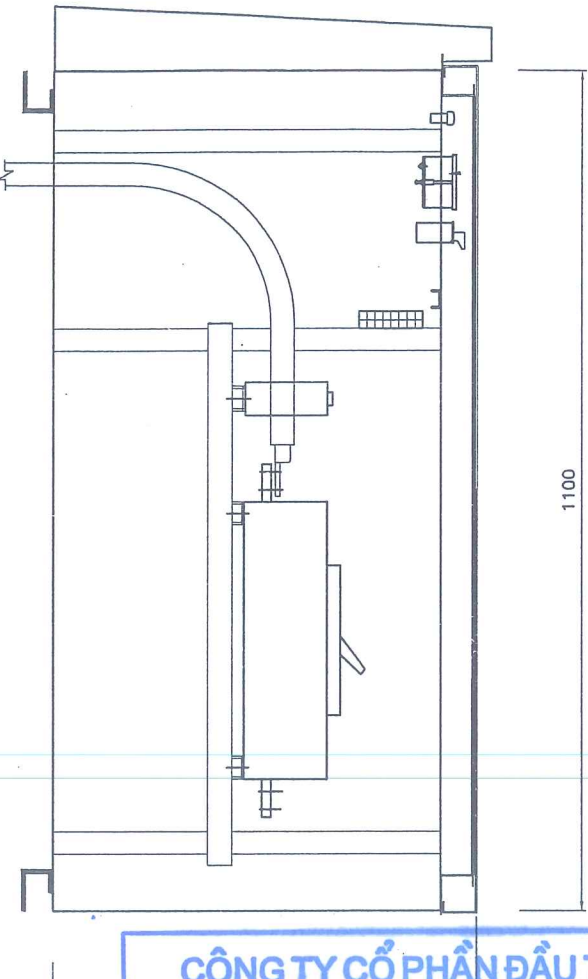
MẶT CẮT II-II
