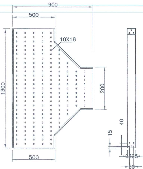
CHI TIẾT CÚT TN1 MÁNG CÁP 200X100
