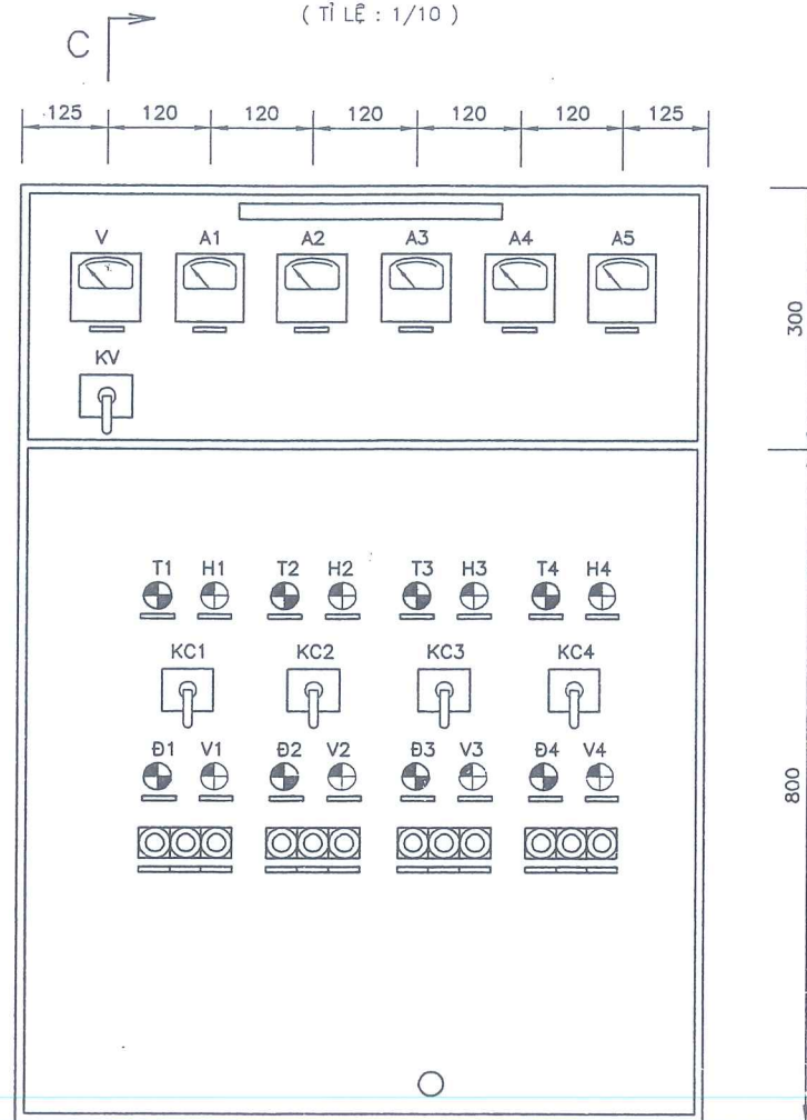
NHÌN THEO A-B (TỈ LỆ: 1/10)
