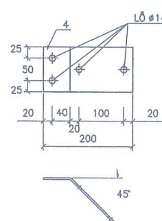
CHI TIẾT 4
