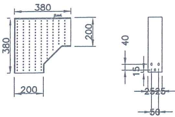
CHI TIẾT TREO MÁNG CÁP
