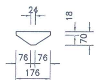
MIẾNG ỐP GÓC ④
