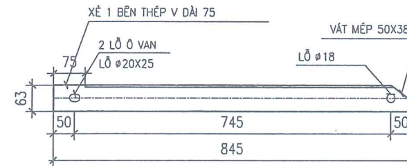
CHI TIẾT THANH CHỐNG ②A TỶ LỆ 1:10
