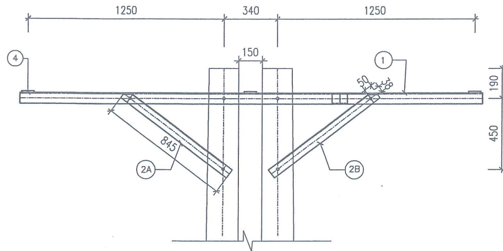
HÌNH CHIẾU BẰNG TỶ LỆ 1:25
