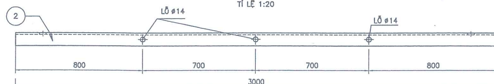
MẶT ĐỨNG CHỐNG SÉT VAN
