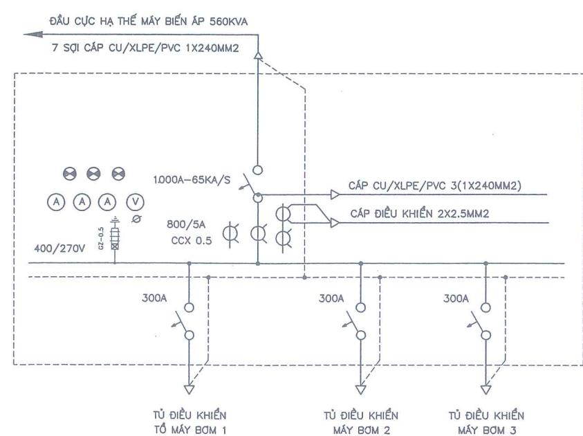
SƠ ĐỒ NỐI ĐIỆN CHÍNH CỦA TỦ MBA 560KVA
