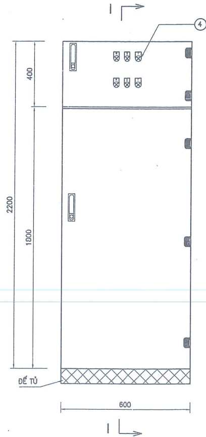
MẶT TRƯỚC TỶ LỆ: 1/20
