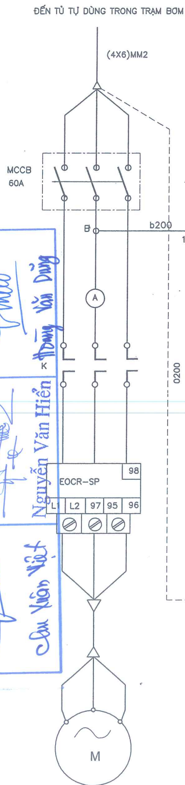
ĐỘNG CƠ CHO BƠM MỖI 7.5KW-380V
