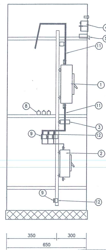
MẶT CẮT I-I TỶ LỆ: 1/20
