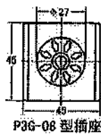
P3G-08 型插座
