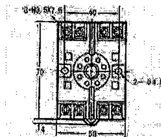
装置式及导轨式插座 P2CF-08 型 (选配件)
