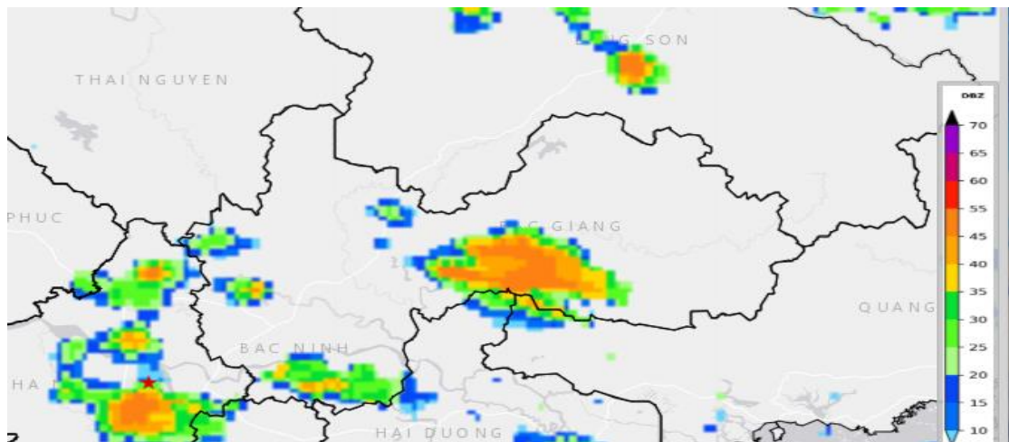
Hình 1: Ảnh radar thời tiết tỉnh Bắc Ninh. (Nguồn: Trung tâm Kỹ thuật quan trắc khí tượng thủy văn, http://hymetnet.gov.vn )
