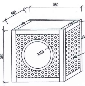
RỌ TRONG
