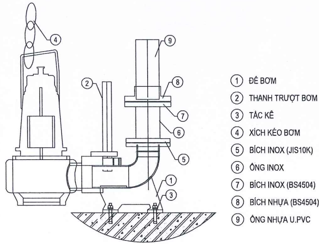
CHI TIẾT LẮP ĐẶT ĐỂ BƠM CHÌM
