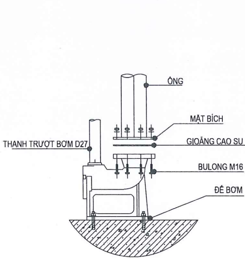
CHI TIẾT LẮP ĐẶT ĐỂ BƠM
