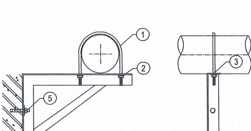
CHI TIẾT GIÁ ĐỠ ỜNG THÀNH BỀ
