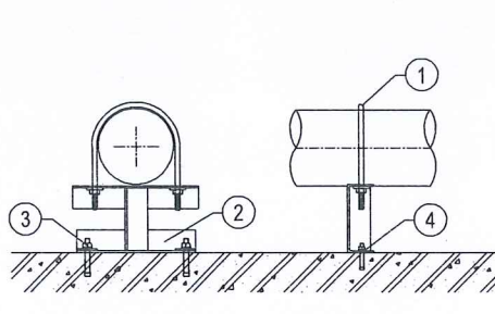
CHI TIẾT GIÁ ĐỠ ỜNG MẶT BỀ (NGOÀI BỀ)
