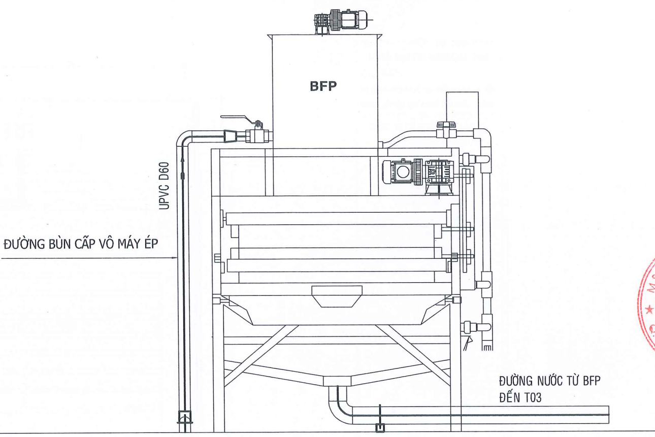
HƯỚNG NHÌN 6-6
