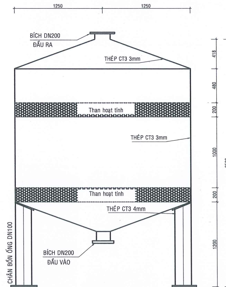
MẶT CẮT 2-2
