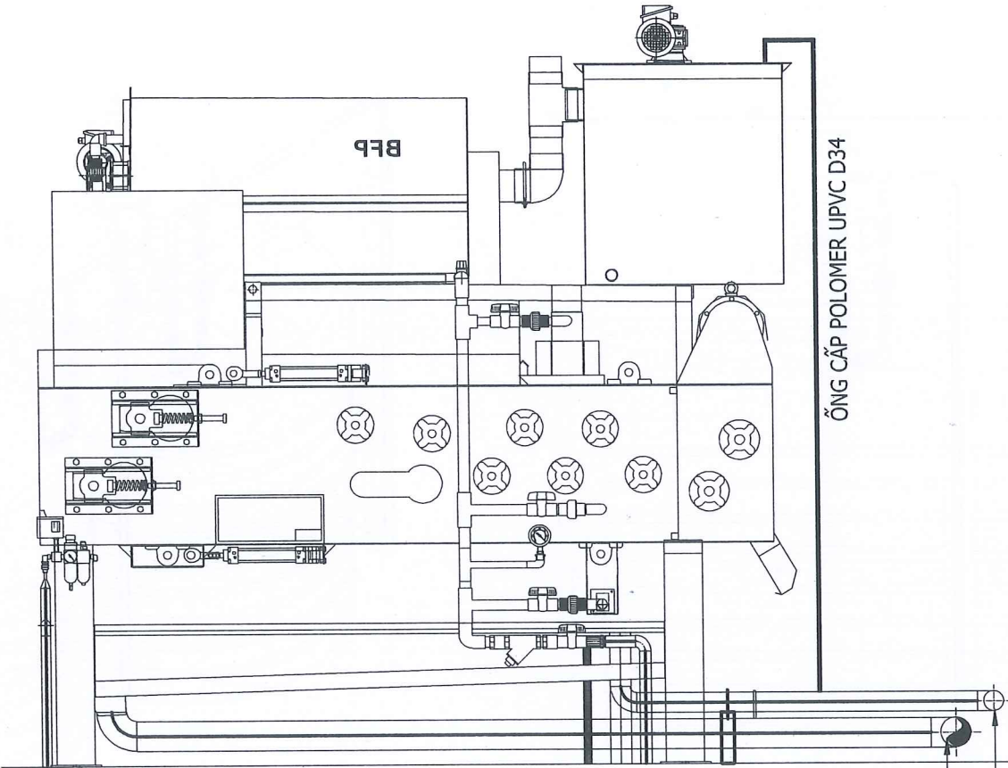
HƯỚNG NHÌN 3-3
