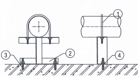
CHI TIẾT GIÁ ĐỠ ỜNG MẶT BỀ (TRONG BỀ)
