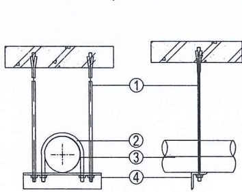
CHI TIẾT GIÁ TREO ỜNG TREO TRẦN BỀ
