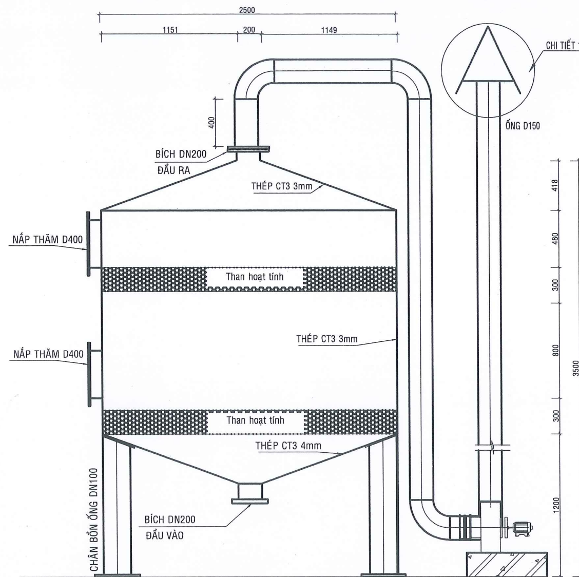
MẶT CẮT 1-1
