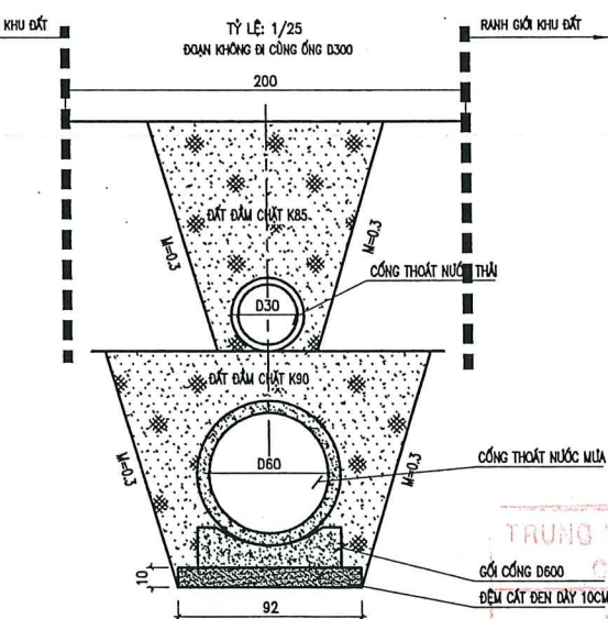
MẶT CẮT ĐIỂN HÌNH CỐNG D600 NGẦM ĐOẠN QUA CỐNG THOÁT THẢI D300
