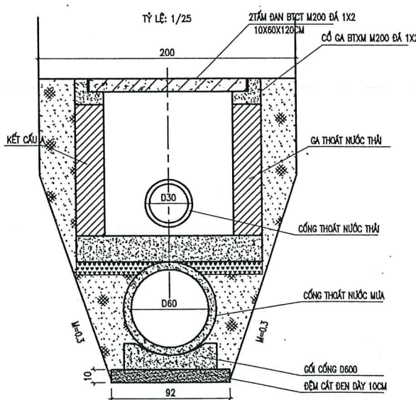
MẶT CẮT ĐIỂN HÌNH CỐNG D600 NGẦM ĐOẠN QUA GA THOÁT THẢI
