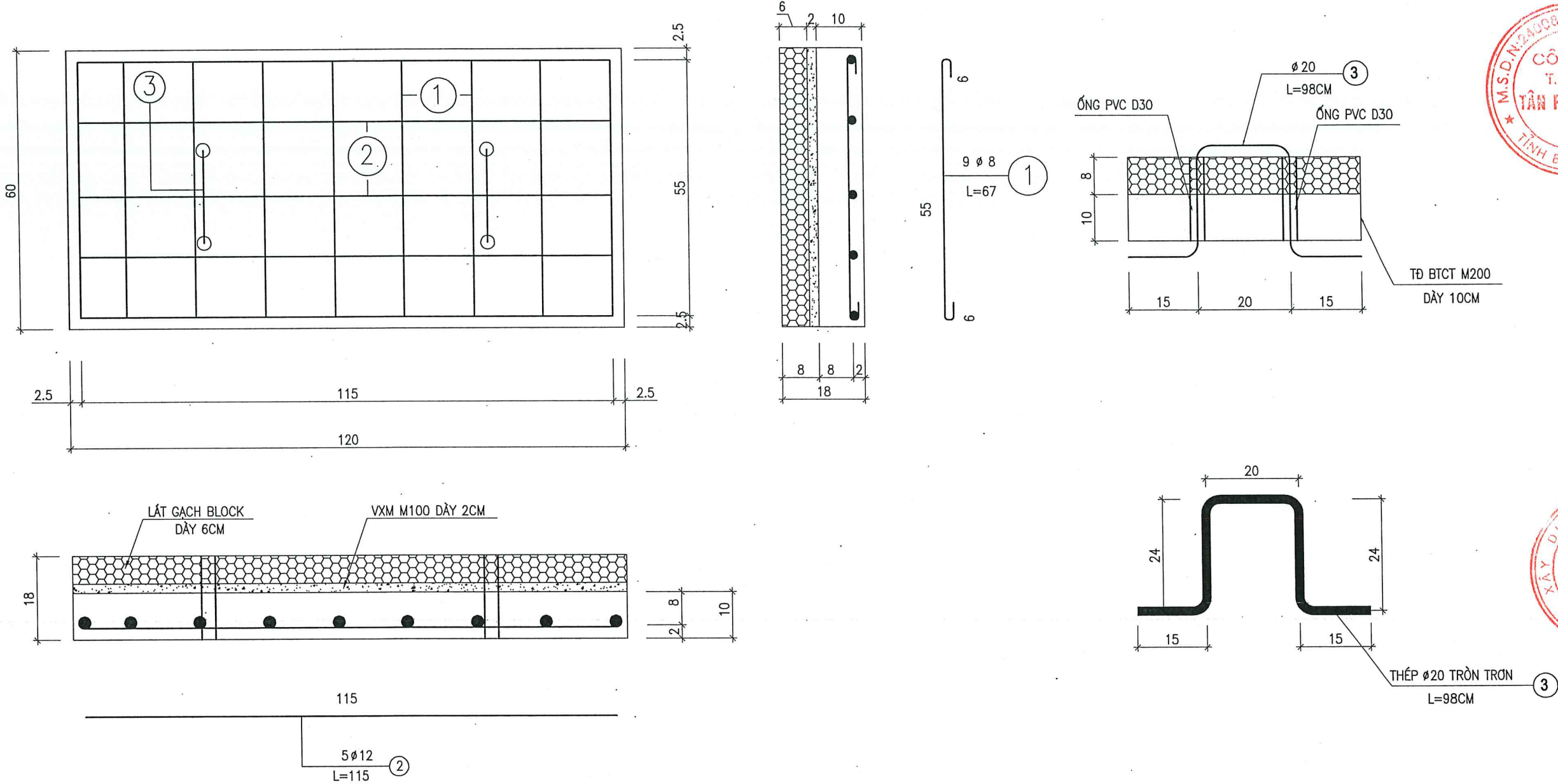
BẢNG THỐNG KÊ CỐT THÉP TẦM ĐƠN HỒ GA CHO 1 TẦM ĐƠN
