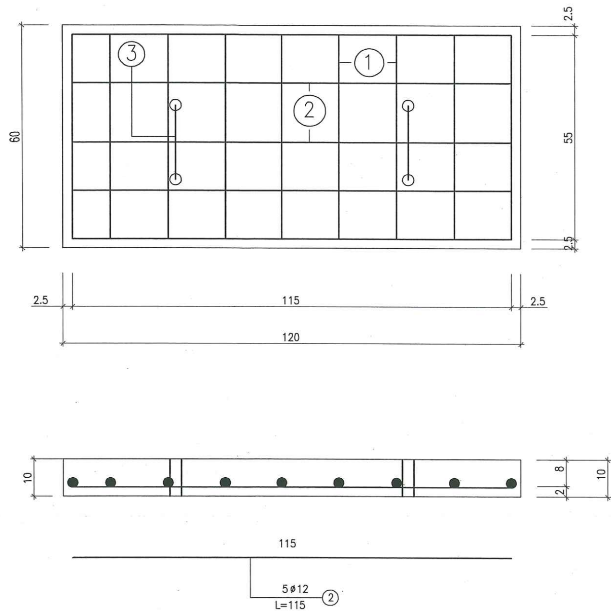
BẢNG THỐNG KÊ CỐT THÉP TẤM ĐẠN HỐ GA CHO 1 TẤM ĐẠN
