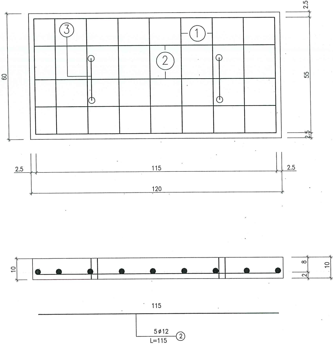
BẢNG THỐNG KÊ CỐT THÉP TẤM ĐAN HỐ GA CHO 1 TẤM ĐAN
