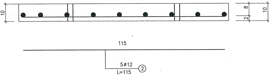
BẢNG THỐNG KÊ CỐT THÉP TẤM ĐAN HỔ GA CHO 1 TẤM ĐAN
