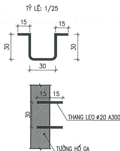
CHI TIẾT THÉP LEO
