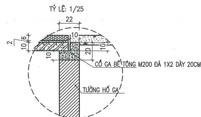
CHI TIẾT B
