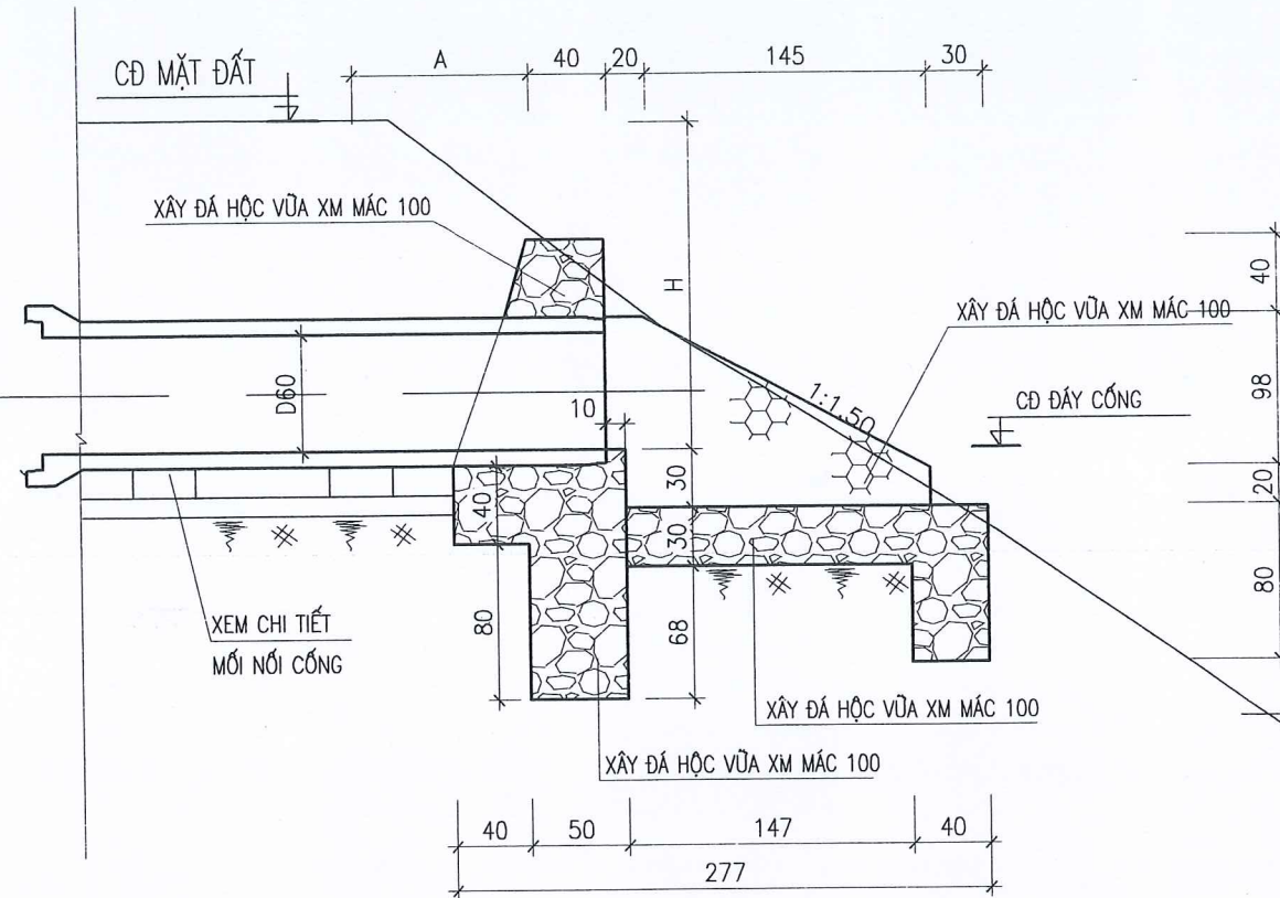
MẶT CẮT 1-1
