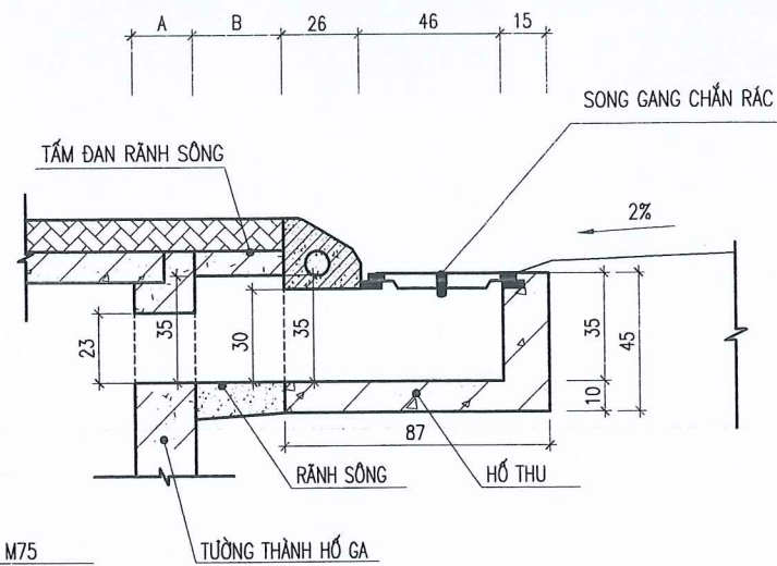
MẶT CẮT 1-1
