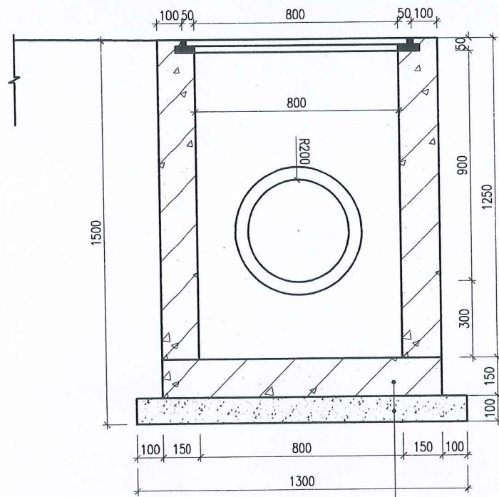
MẶT CẮT 2-2
