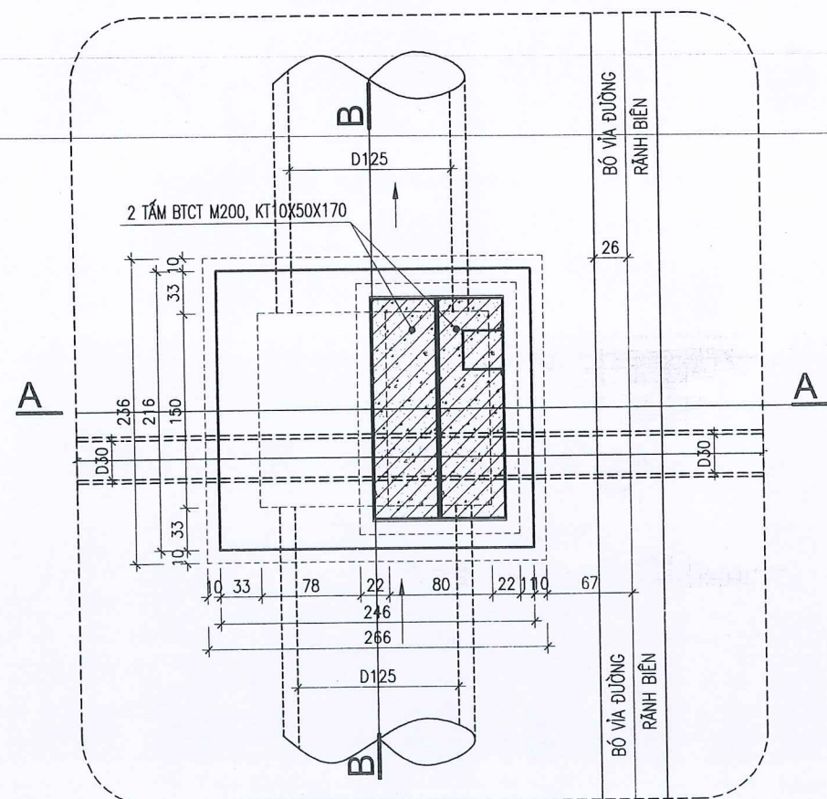
MẶT BẰNG
