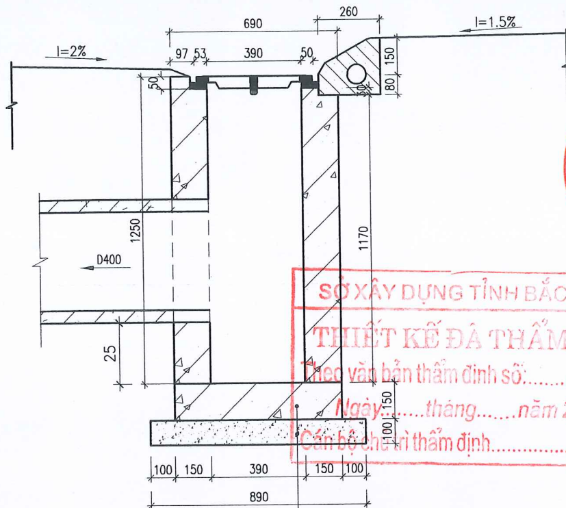
MẶT CẮT 1-1
