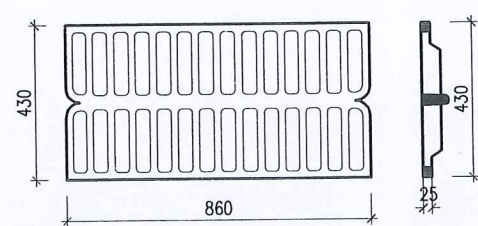
MẶT BẰNG
