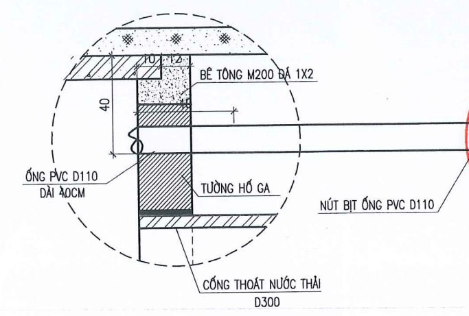
CHI TIẾT ỐNG PVC
