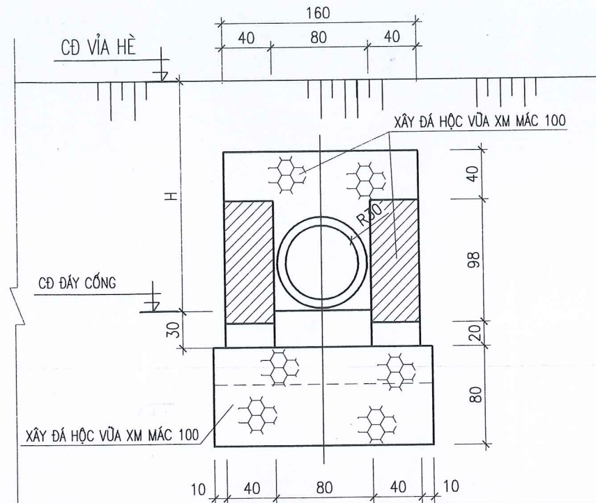
MẶT ĐỨNG CỦA XẢ
