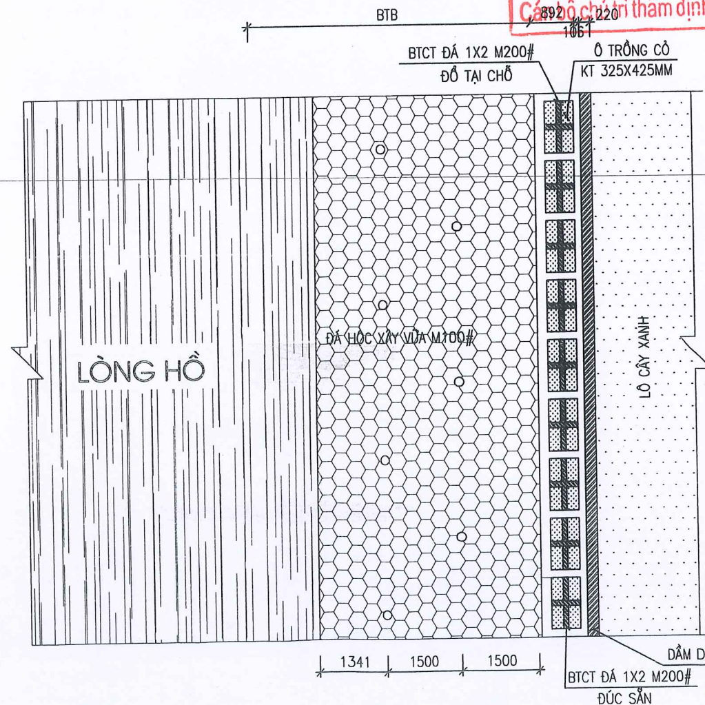
MẶT BẰNG KÈ BỜ HỒ
