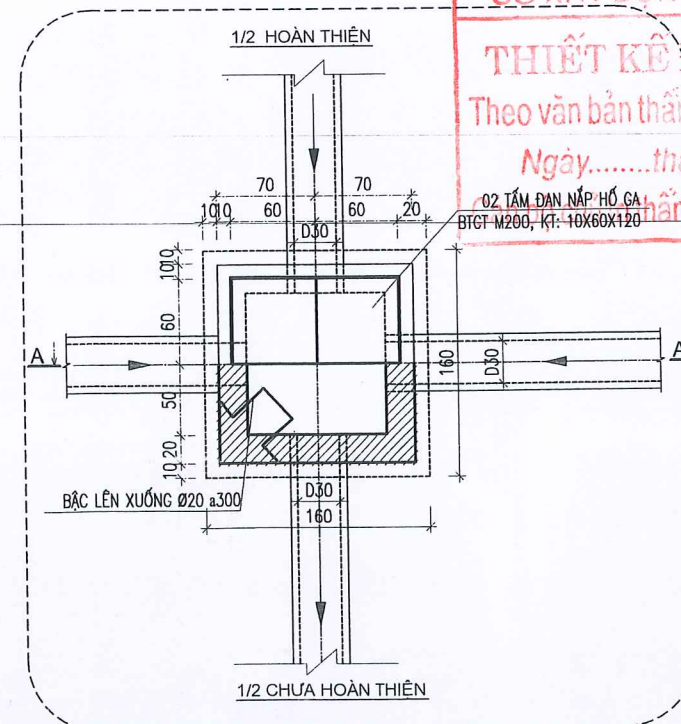
MẶT BẰNG
