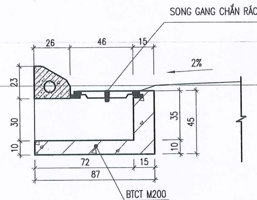
MẶT CẮT 1-1
