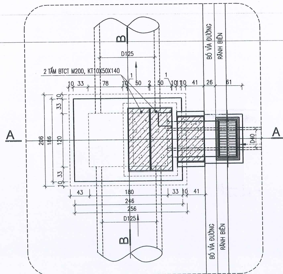
MẶT BẰNG
