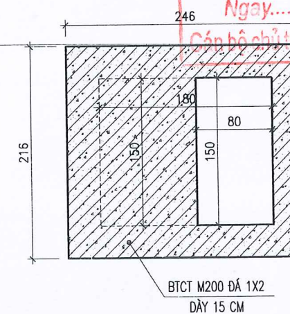
BÊ TÔNG SÀN HỒ GA
