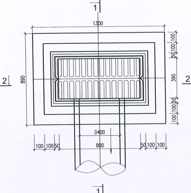
MẶT BẰNG
