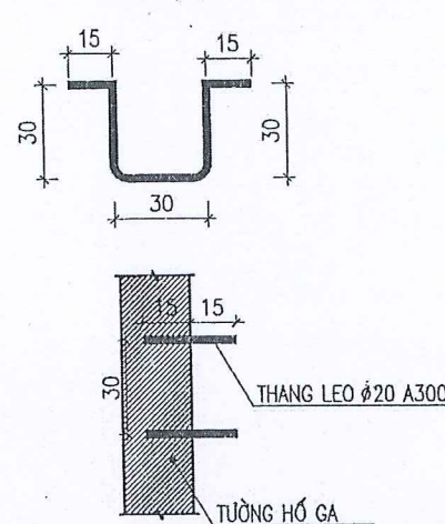
CHI TIẾT THÉP LEO
