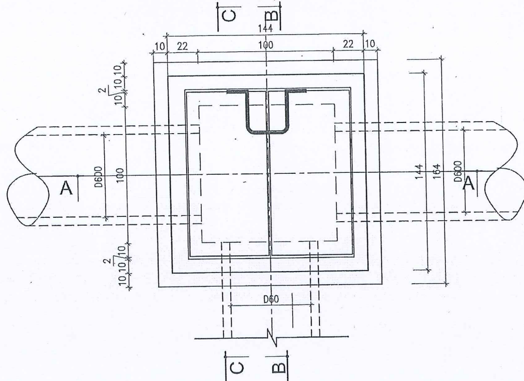
MẶT BẰNG
