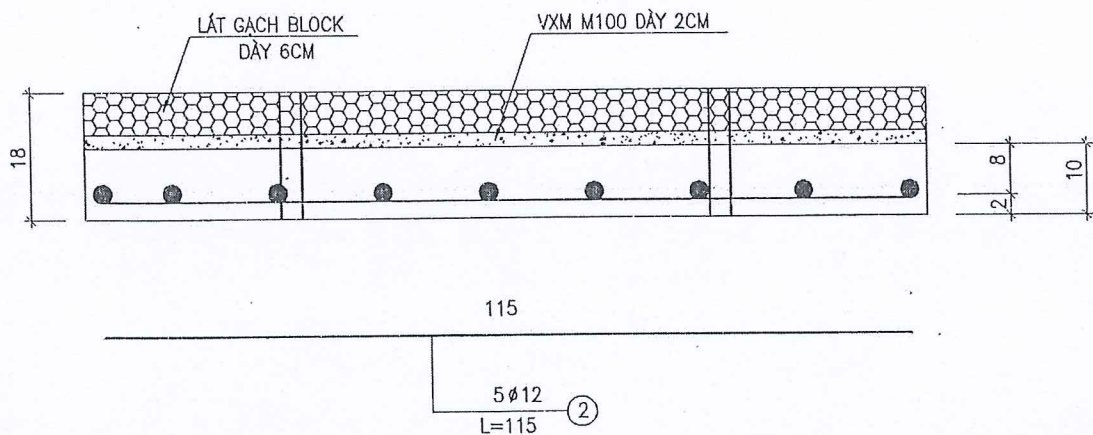
BẢNG THÔNG KÊ CỐT THÉP TẤM ĐẠN HỔ GA CHO 1 TẤM ĐẠN
