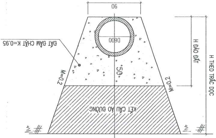
MẶT CẮT MƯƠNG ĐÀO CÔNG D600
