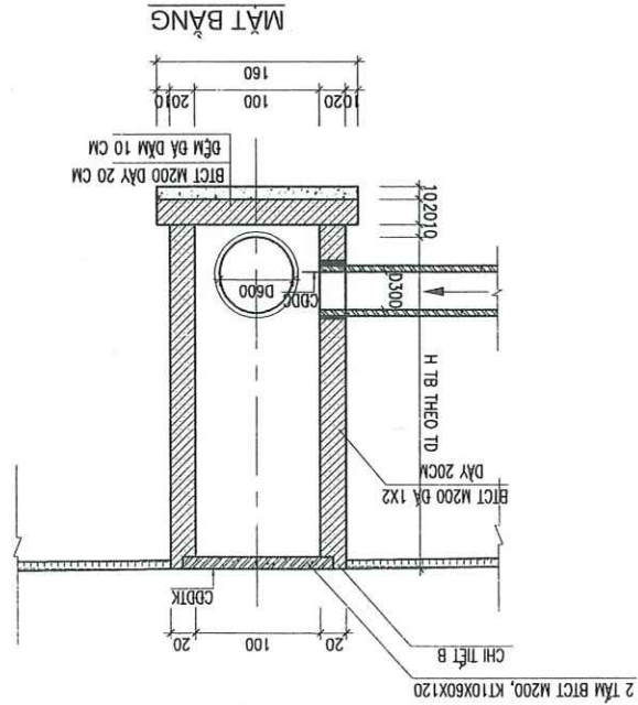
KIỂU CẦU TẠO HỒ GÀ KIỂU 8
