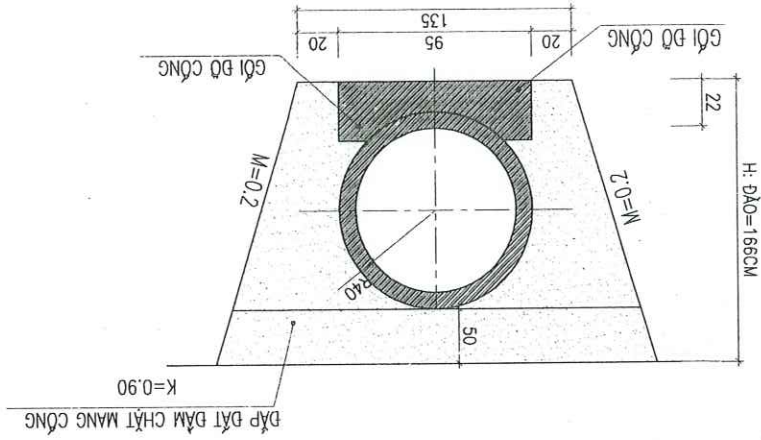
MẶT CẮT MƯƠNG ĐÀO CÔNG D800 TRÊN HỀ
