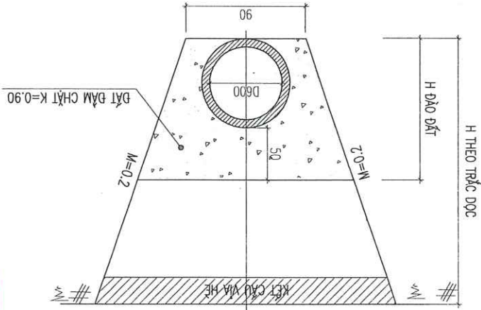
MẶT CẮT MƯƠNG ĐÀO CÔNG D600
