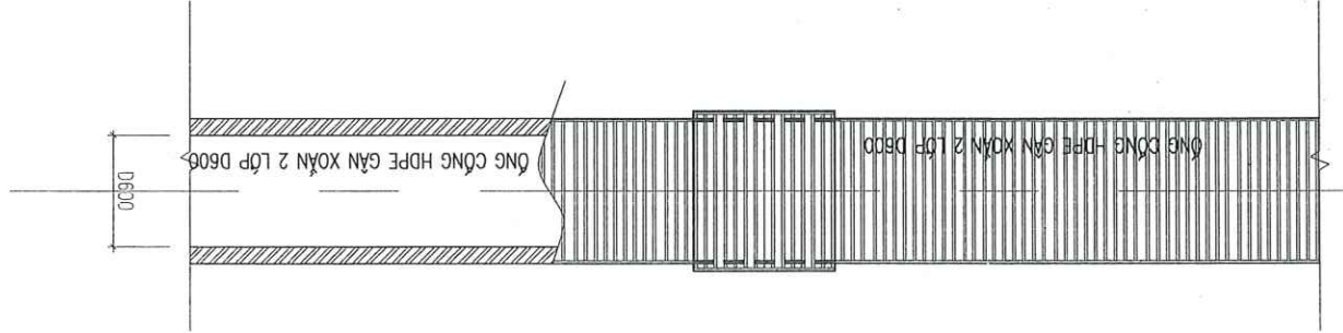
CHI TIẾT LẬP GHEP VÀ NỐI CÔNG D600
